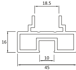
Top & Bottom Profile : Code : BWAY-TB-4516
