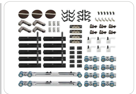
BWAY-MW-5-Slide Door Max Door Width : 900 mm
