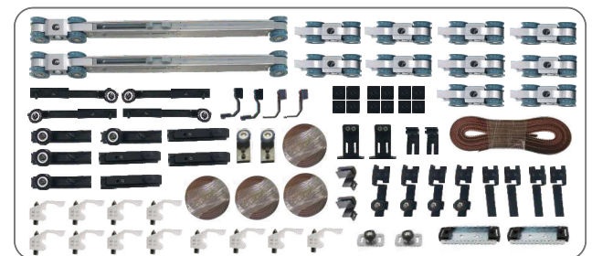
BWAY-TLS+SYN 2+6 (2 Fix + 6 Door Sliding)
